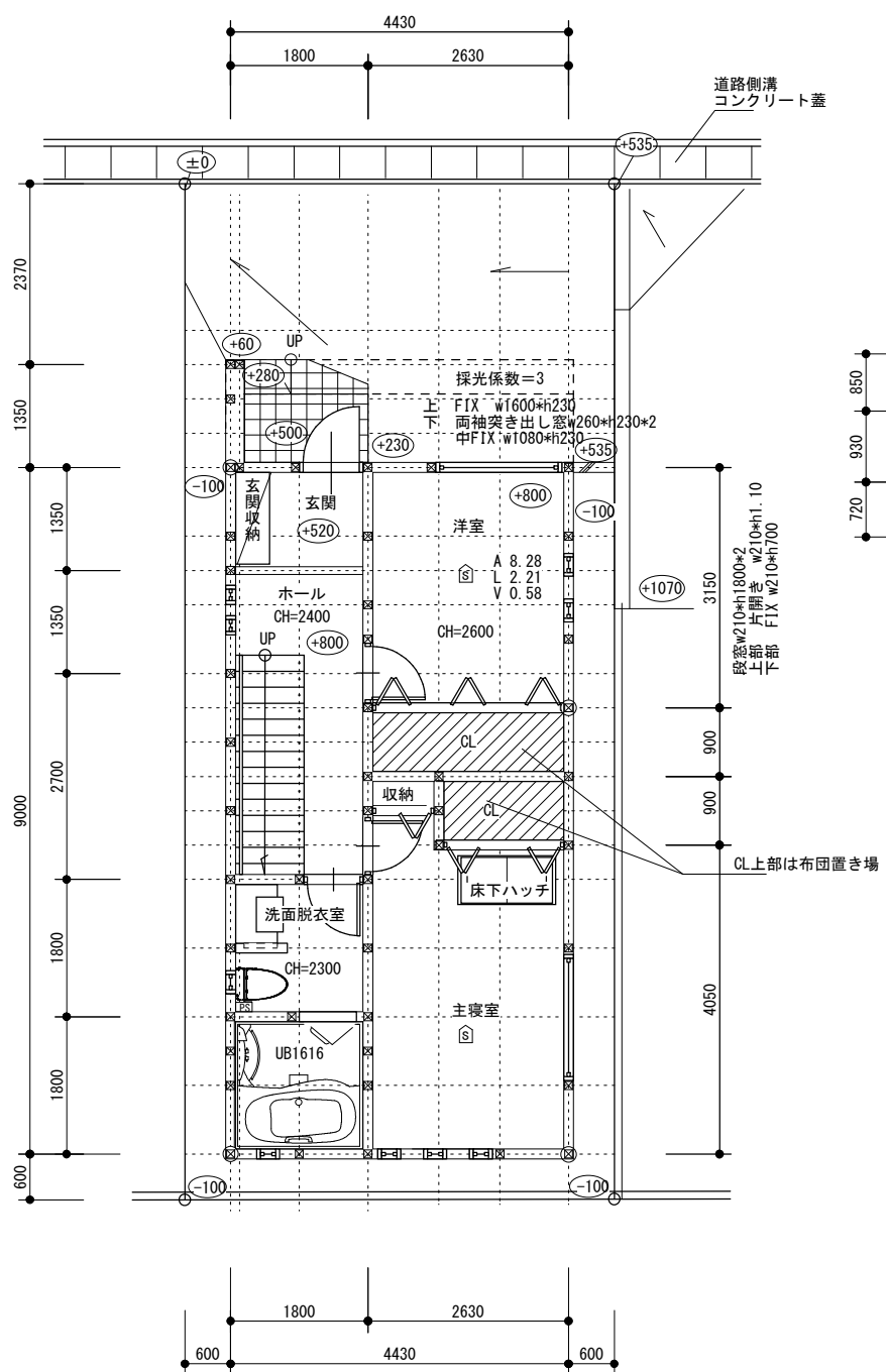
1階平面図
